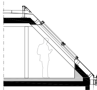
SCHNITT 1-1
